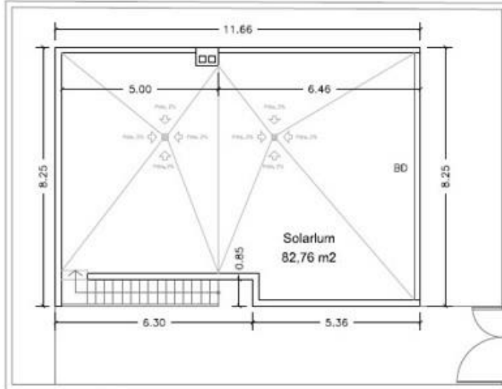
Solarium
